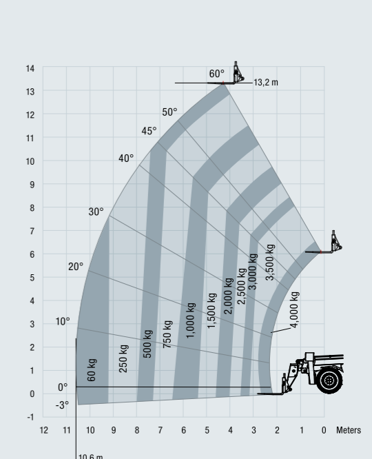
STH1840 – STABILIZZATORI ESTESI E APPOGGIATI STH1840 – STABILIZZATORI SOLLEVATI
