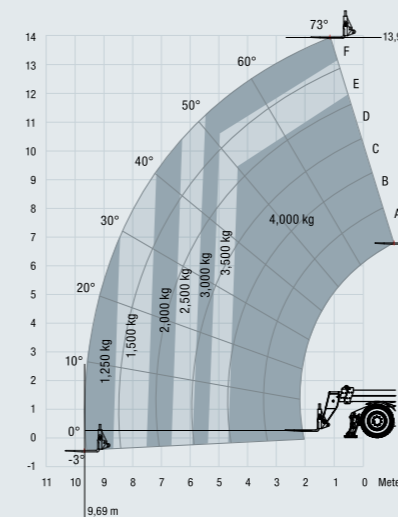
STH1840 – STABILIZZATORI ESTESI E APPOGGIATI STH1840 – STABILIZZATORI SOLLEVATI
